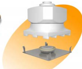
Bulk Tablet IBC and Tablet Discharge Station 錠剤用IBC 錠剤用排出ステーション
